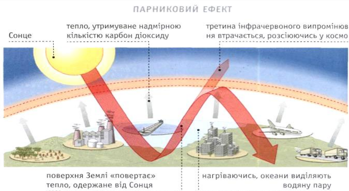
Рис. 7.3. Парниковий ефект [29]
